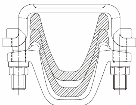
Spoj s horním unášečem
